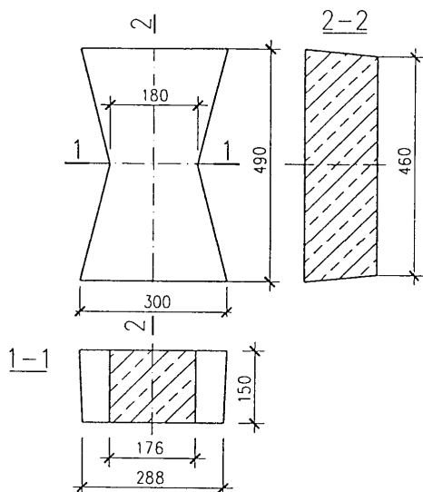
DYBEL DC-15
