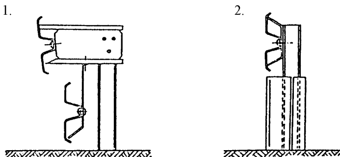
Załącznik 11.5. Dodatkowe urządzenia zabezpieczające użytkowników pojazdów jednośladowych na łukach drogi, wg [32]
