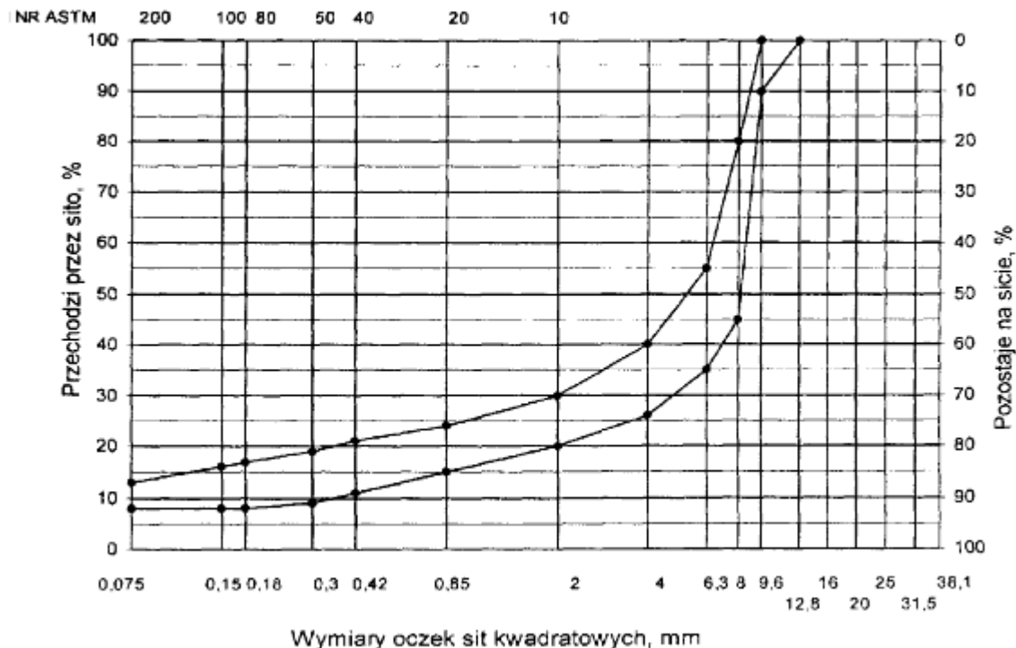
Rysunek 1 Krzywe graniczne uziarnienia mieszanki mineralnej SMA od 0 do 9,6 mm do warstwy ściernalnej nawierzchni drogi o obciążeniu ruchem KR1 lub KR2
