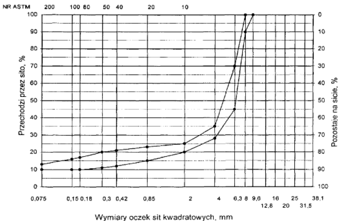
Rysunek 7 Krzywe graniczne uziarnienia mieszanki mineralnej SMA od 0 do 8 mm do warstwy ścieralnej nawierzchni drogi o obciążeniu ruchem od KR3 do KR6
