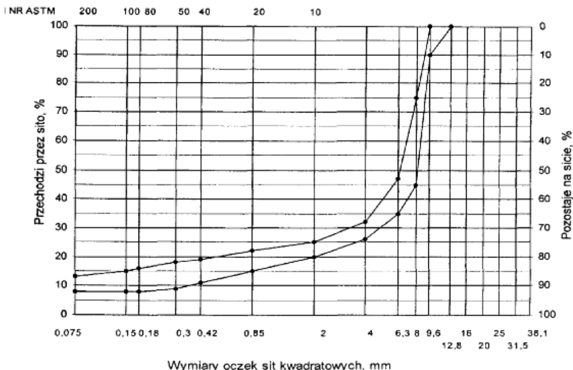
Rysunek 6 Krzywe graniczne uziarnienia mieszanki mineralnej SMA od 0 do 9,6 mm do warstwy ścieralnej nawierzchni drogi o obciążeniu ruchem od KR3 do KR6
