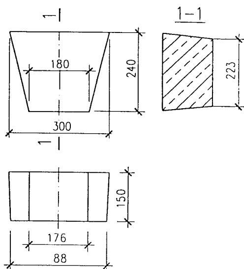
DYBEL DP-15
